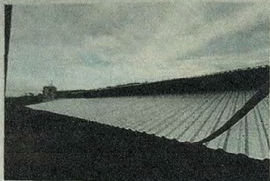
Foto 1. Sustitución de lamina, por lamina troquelada aluzinc en el modulo 1
